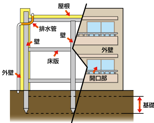
鉄筋コンクリート造の例
